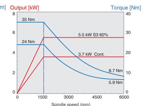
Live tool spindle motor
